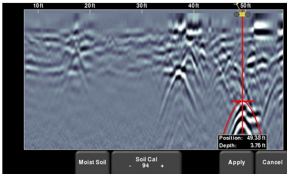
图 8-11: 当处于后退模式时调整土壤标定值
