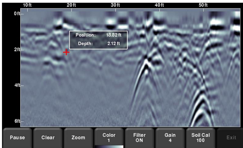
图 8-4：触摸屏获得任意点的深度和水平位置
