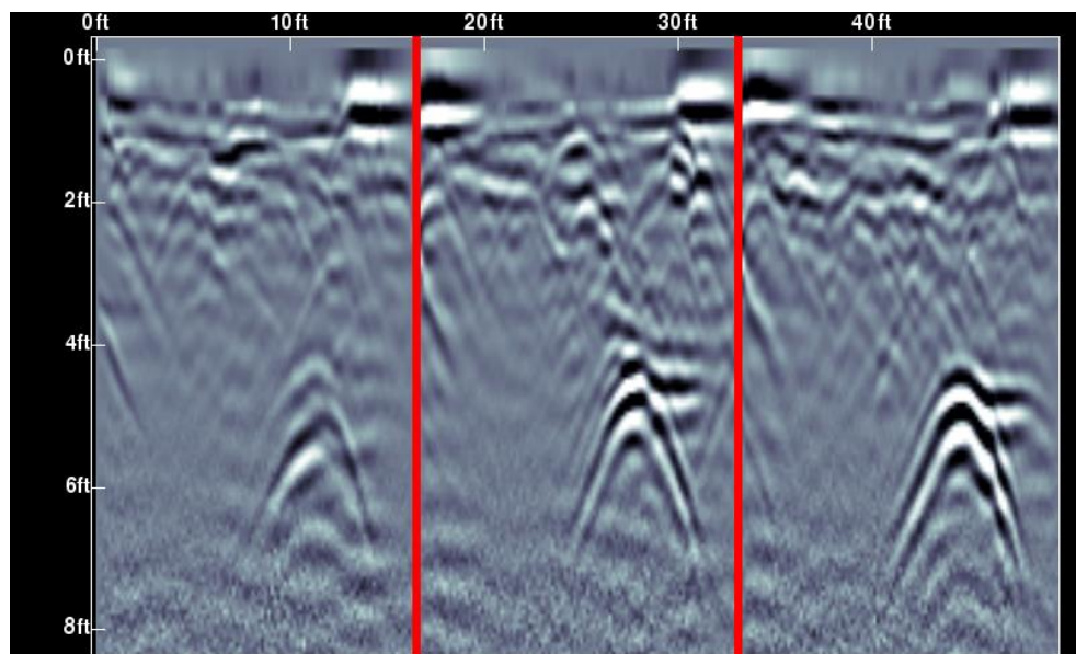
图 8-13: 按暂停然后恢复数据收集。
