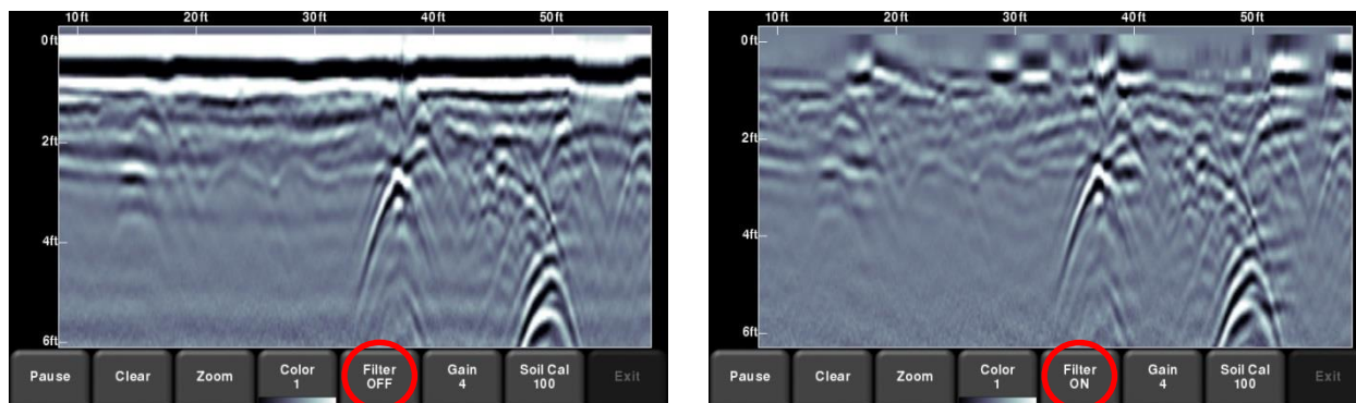
图 8-10: 左侧的图片是滤波器设为关闭 (Off) 时的数据图像, 右侧则是相同的数据在滤波器设为开启 (On) 时所呈现的图像
