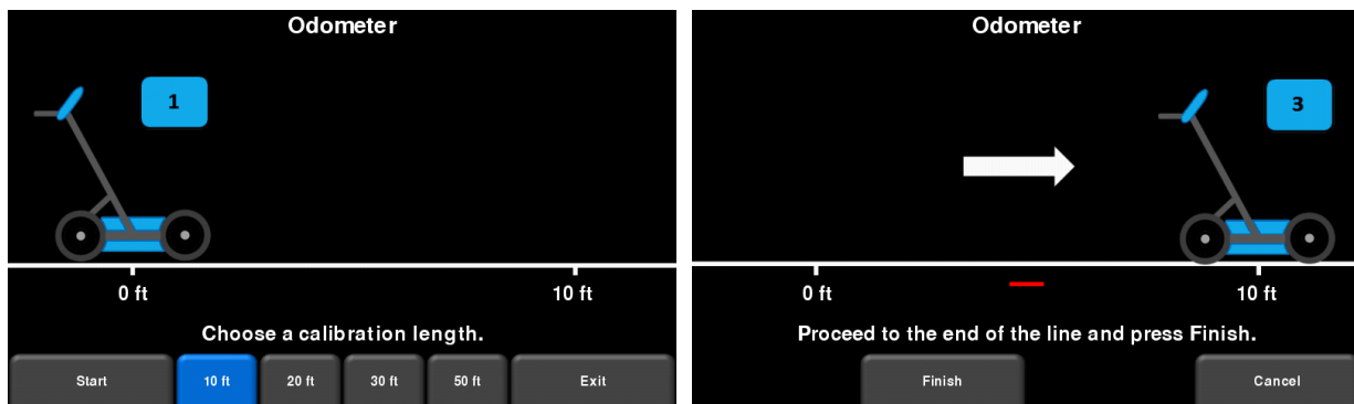
图 6-13: 里程表测试。左侧的图片显示用户必须选择一个距离的屏幕。右边的图片指导您移到该距离然后按 完成 (Finish) 。
