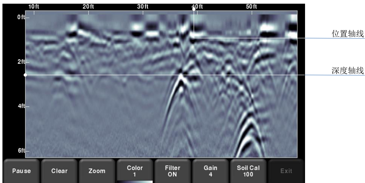
图 8-2: 线扫描采集模式, 显示收集的数据和轴线标签
