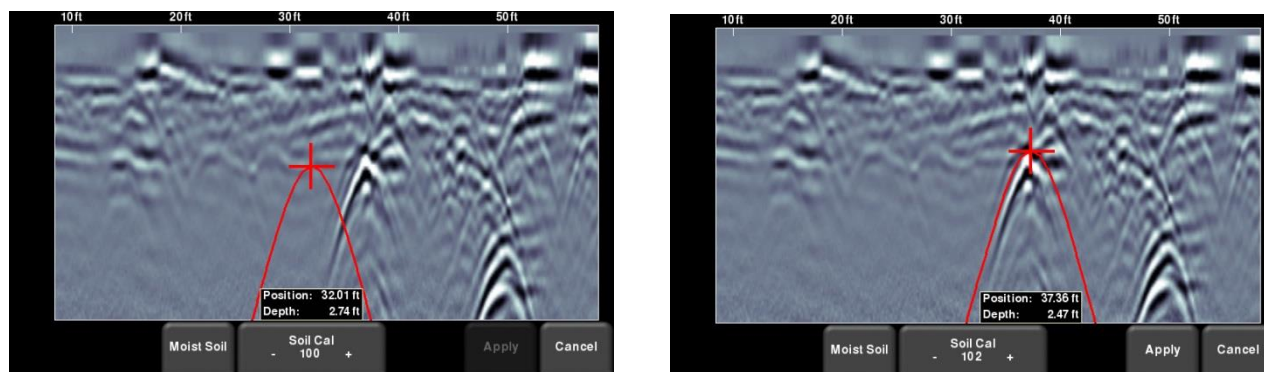
图 8-12: 按 土壤标定值 (Soil Cal) 显示一条红色双曲线 (左边)。然后移动双曲线，使其位于来自地面的一条双曲线的上方然后调节形状 (右边)
