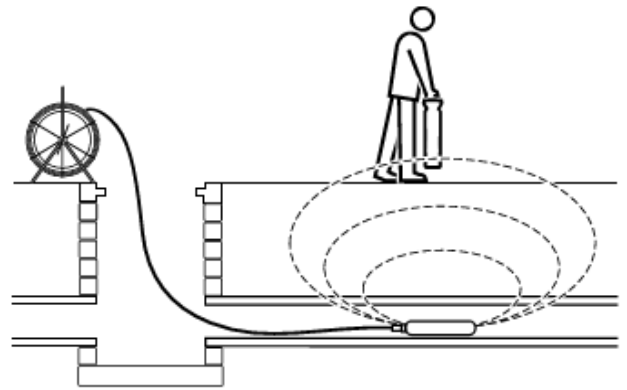
Figuur 9.7 Sonde-installatie
