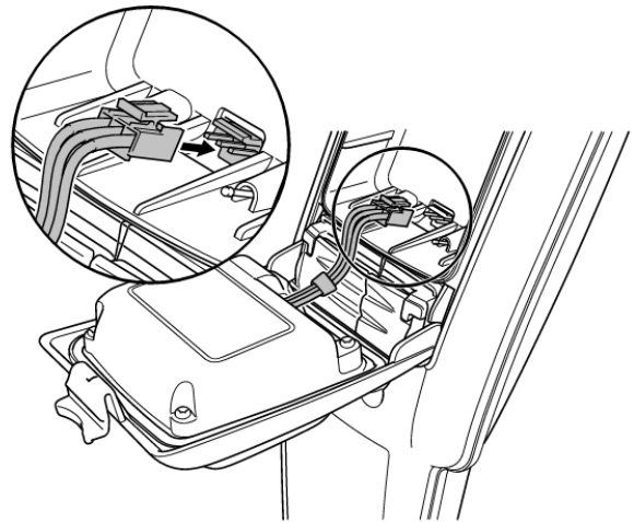
Afbeelding 4.7 De Li-Ion stekker aansluiten
