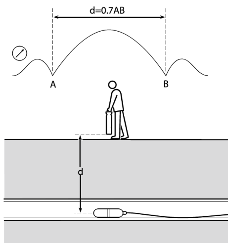
Figuur 9.9: Sondediepte berekenen
