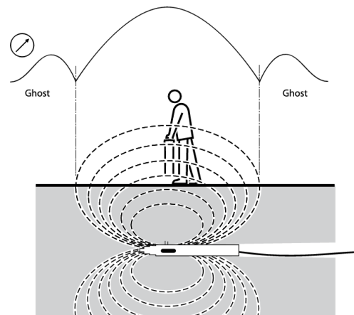
Figuur 9.8 Een sonde lokaliseren
