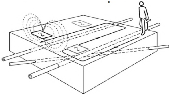
Figuur 5.6 Uitnullen – één persoon
