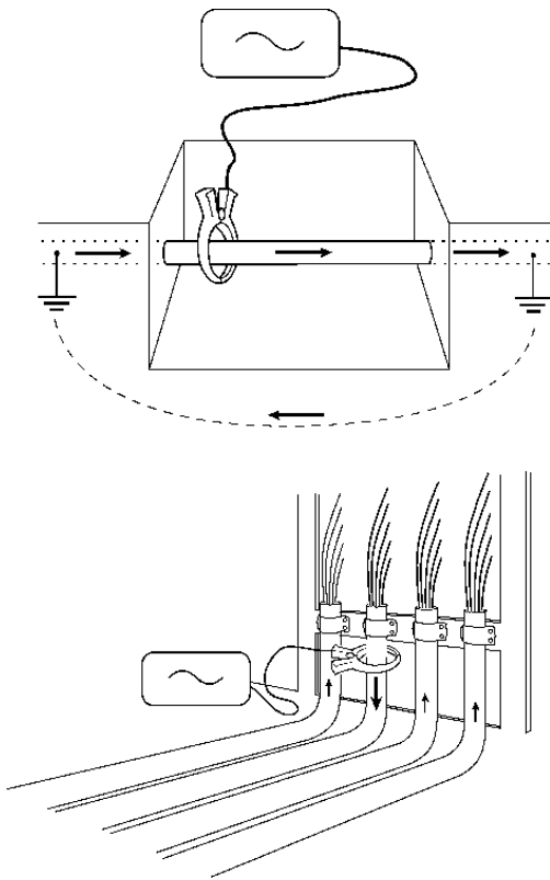
Figuur 9.5 - 9.6: Zendtangen aansluiten
