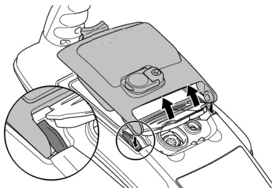
Figura 4.6 Instalación de baterías nuevas
