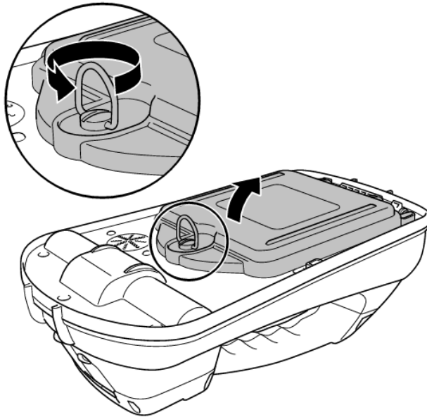
Figura 4.9: Apertura del compartimiento de la batería.
