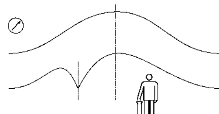
Figura 5.3: Señalización con indicadores Pico y Nulo
