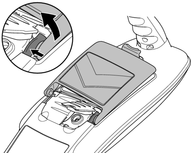
Figura 4.5 Repita y levante la batería para extraerla
