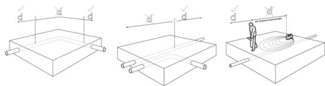
Figura 6.2: Lecturas de profundidad
