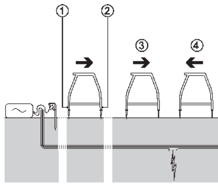
Figura 8.1: Búsqueda de fallos en el revestimiento de cables
