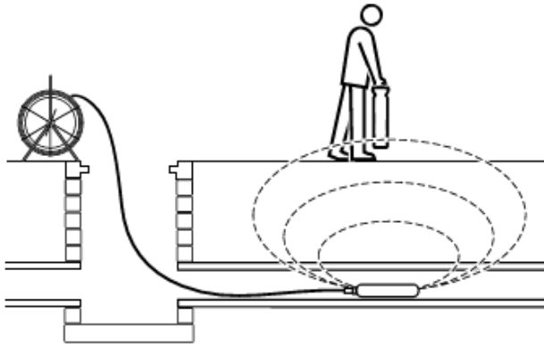
Figura 12.10 Despliegue de una sonda
