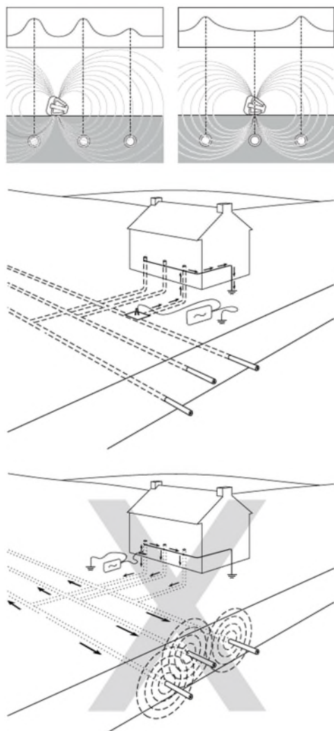
Figuras 7.1 – 7.4: Anulación de servicios e interferencia de los servicios
