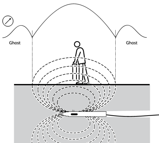
Figura 12.11 Localización de una sonda
