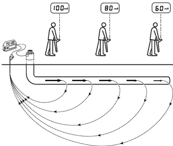
Figura 6.7: Lecturas de corriente usando señales del transmisor
