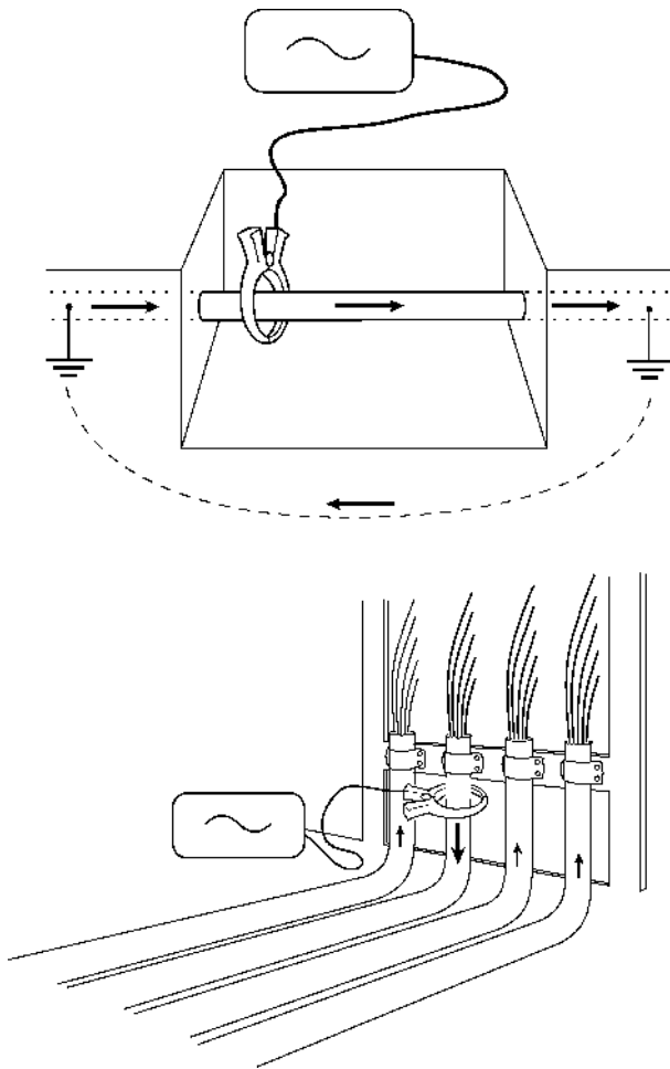
Figuras 12.5: – 12.6.: Conexión de pinzas de transmisor
