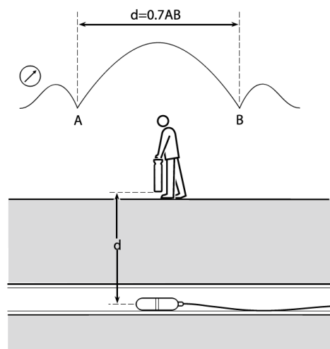
Figura 12.12: Cálculo de la profundidad de la sonda
