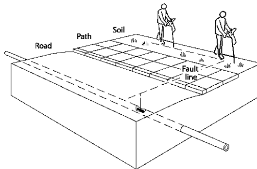
Figura 8.2: Localización de fallos con el localizador y el A-Frame
