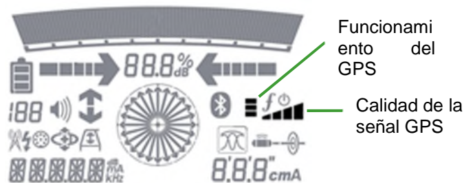
Figura 4.14 Iconos de GPS
