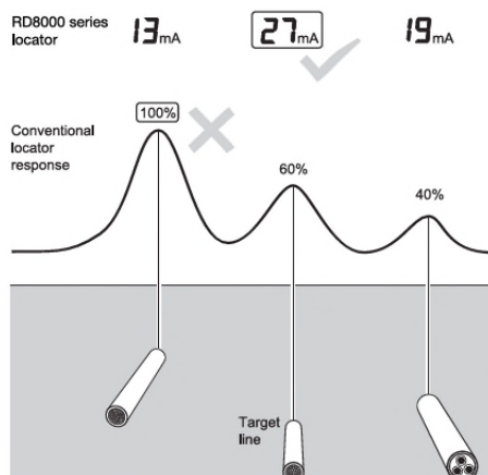
Figuras 6.4 – 6.6 Toma de lecturas de corriente
