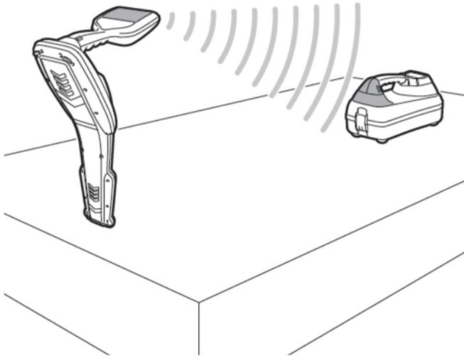
Figura 11.1 Uso de iLOC
